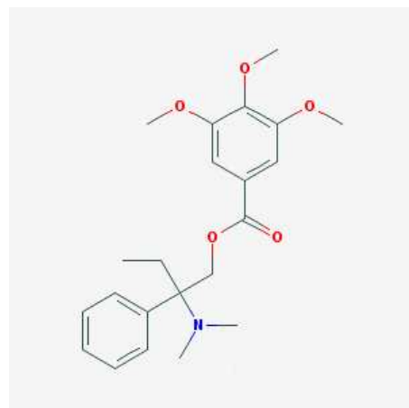
그림 1. 트리메부틴의 구조식
