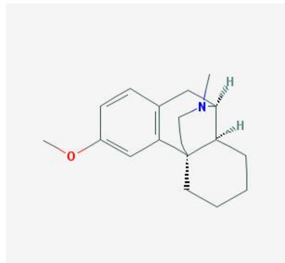
그림 1. 덱스트로메토르판의 구조식
